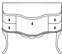
МО 386 L 106 P 58/41 H 82 один ящик четыре ящичка
