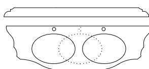
РОМА195 для 1 встроенной РОМА295 для 1 встраиваемой РОМА196 для 2 встроенных РОМА296 для 2 встраиваемых L 167/149 P 59 H 2
