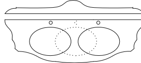
ROMA184 для 1 встроенной ROMA284 для 1 встраиваемой ROMA186 для 2 встроенных ROMA286 для 2 встраиваемых L 177/148 P 65 H 2
