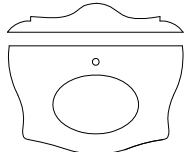
РОМА119 встроенная РОМА219 встраеваемая L 91/77 P 59 H 2
