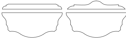
РОМА105 L 135/115 P 67 H 2 РОМА106 L 135/115 P 67 H 2
