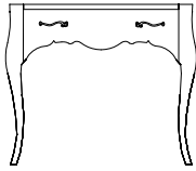
MO 278 L 115/95 P 58 H 83 один ящик
